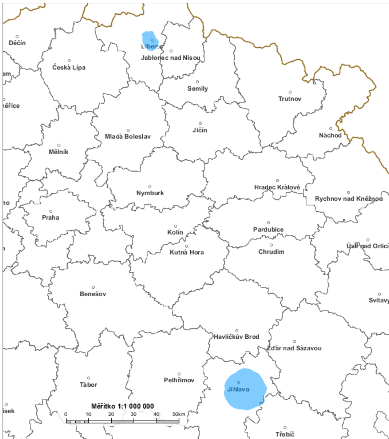
Diagram využití rádiových kmitočtů určených pro analogové vysílání v pásmu VKV pro vysílače JIHLAVA HOLY VRCH 96,2 MHz a LIBEREC MESTO I 94,1 MHz stanovený výpočtem podle vyhlášky č. 22/2011 Sb. (modrá barva).
