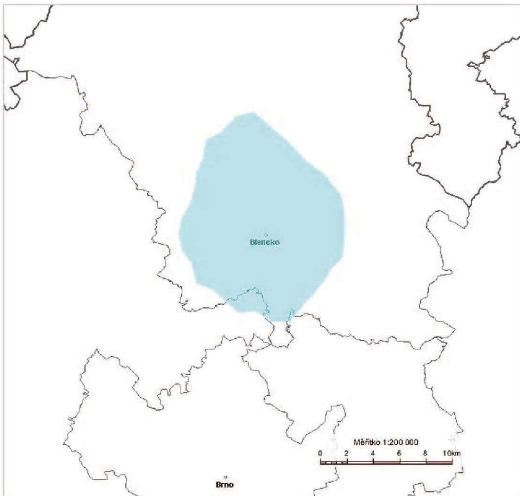
Diagram využití rádiového kmitočtu BLANSKO 3 90,0 MHz stanovený výpočtem podle vyhlášky č. 22/2011 Sb. o způsobu stanovení pokrytí zemského rozhlasového vysílání ve vybraných kmitočtových pásmech – modrá barva.
