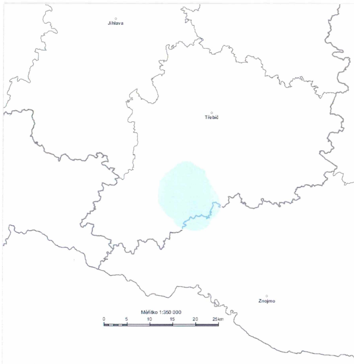
Diagram využití rádiových kmitočtů určených pro analogové vysílání v pásmu VKV pro vysílač MORAVSKE BUDEJOVICE 107,9 MHz, stanovený výpočtem podle vyhlášky č. 22/2011 Sb. (modrá barva).
