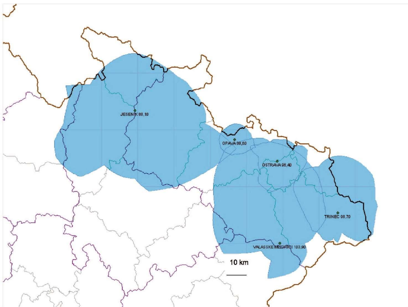
Diagram využití rádiových kmitočtů JESENÍK 88,1 MHz, OPAVA 88,6 MHz, OSTRAVA 96,4 MHz, TRINEC 98,7 MHz a VALASSKÉ MEZIRÍČÍ 103,9 stanovený výpočtem podle vyhlášky č. 22 / 2011 Sb. o způsobu stanovení pokrytí signálem zemského rozhlasového vysílání ve vybraných kmitočtových pásmech – modrá barva.
