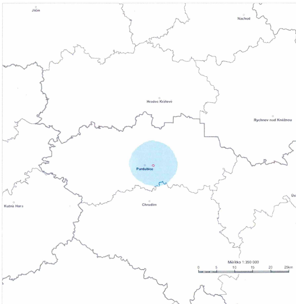
Diagram využití rádiových kmitočtů určených pro analogové vysílání v pásmu VKV pro vysílač PARDUBICE I 88,0 MHz, stanovený výpočtem podle vyhlášky č. 22/2011 Sb. (modrá barva).
