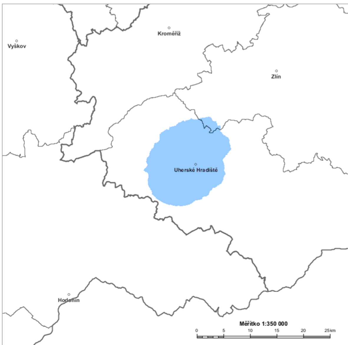
Mapa územního rozsahu překryvu území pokrytého vysílači UHERSKE HRADISTE 7 102,7 MHz (mod) MHz stanovené výpočtem podle vyhlášky č. 22/2011 Sb. o způsobu stanovení pokrytí zemského rozhlasového vysílání ve vybraných kmitočtových pásmech – modrá barva.
