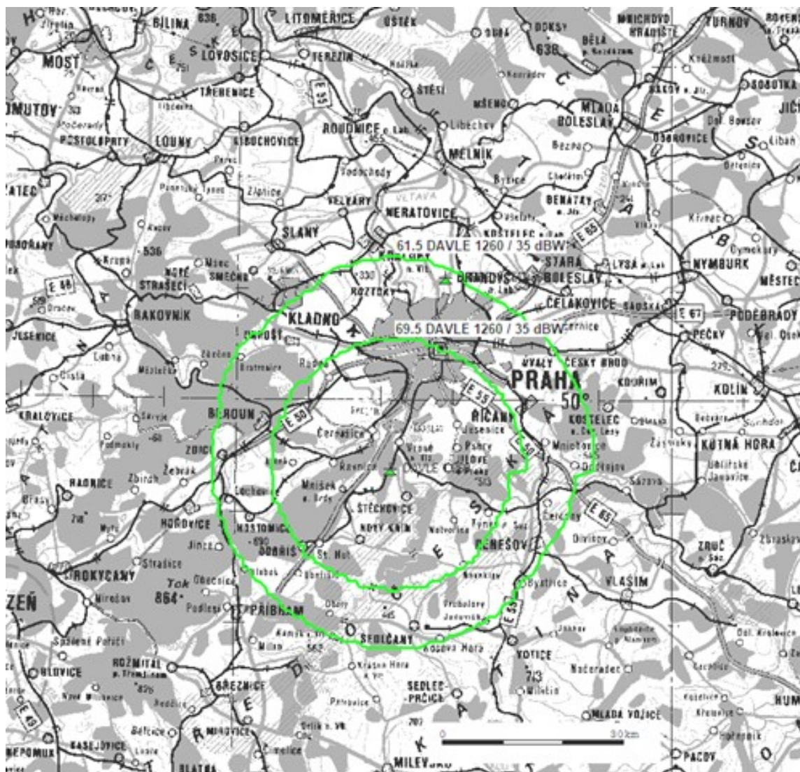
Diagram využití kmitočtu DAVLE 1260 kHz / 37 dBW daný nominální použitelnou intenzitou pole přízemní složky elektromagnetické vlny E_u = 61,5 \text{ dB}_\mu (den, venkov) a 69,5 \text{ dB}_\mu (noc, venkov).
