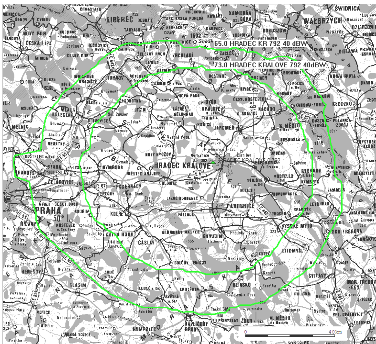
Diagram využití kmitočtu HRADEC 792 kHz / 40 dBW daný nominální použitelnou intenzitou pole přízemní složky elektromagnetické vlny E_u = 65 \text{ dB}_\mu (den, venkov) a 73 \text{ dB}_\mu (noc, venkov).
