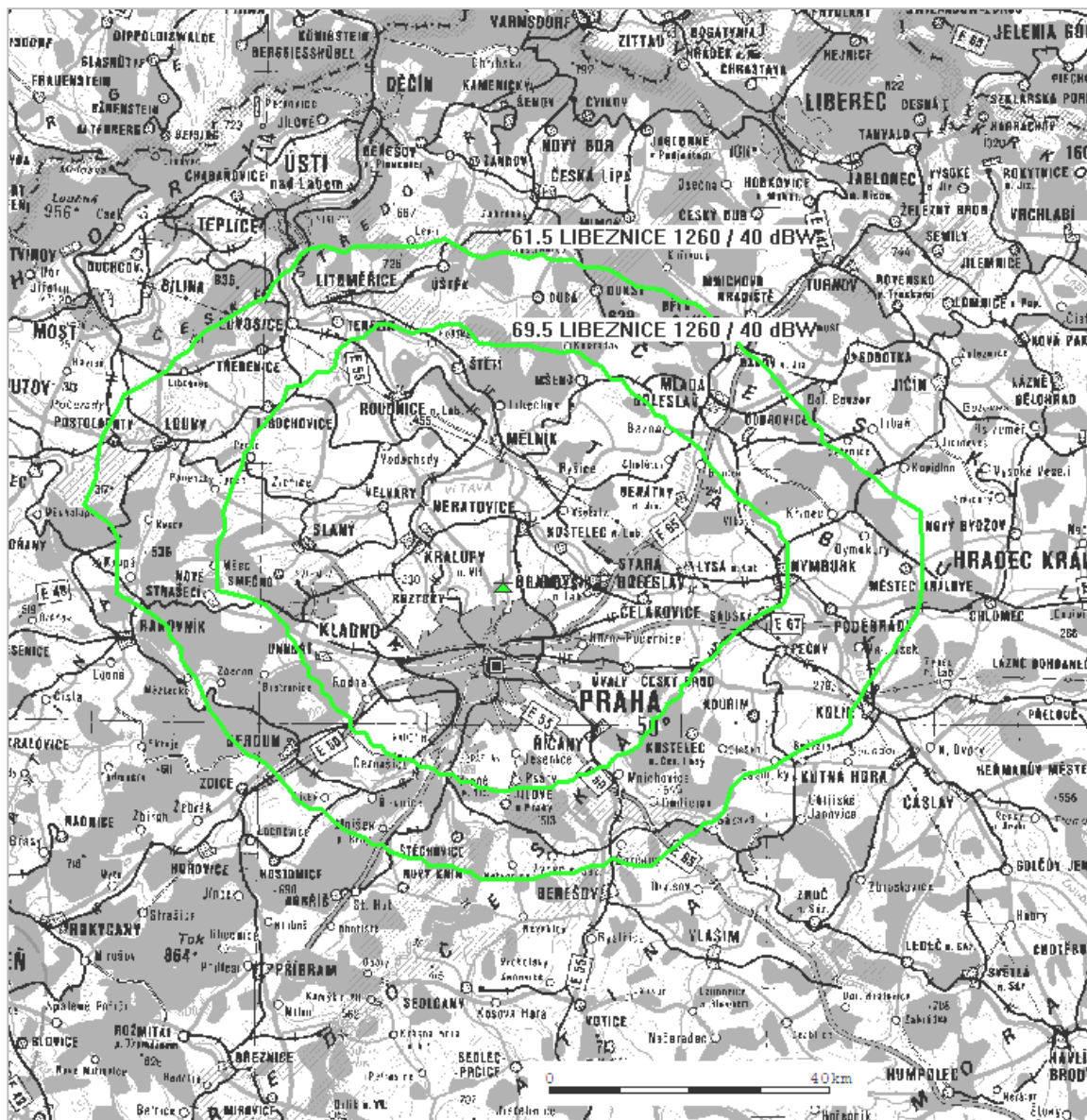
Diagram využití kmitočtu LIBEZNICE 1260 kHz daný nominální použitelnou intenzitou pole přízemní složky elektromagnetické vlny E_u = 61,5 \text{ dB}_\mu (den, venkov) a 69,5 \text{ dB}_\mu (noc, venkov).
