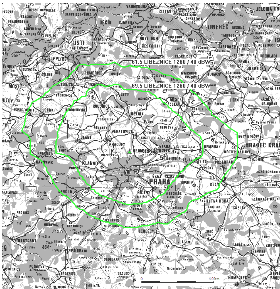
Diagram využití kmitočtu LIBEZNICE 1260 kHz / 40 dBW daný nominální použitelnou intenzitou pole přízemní složky elektromagnetické vlny E_u = 61,5 \text{ dB}_\mu (den, venkov) a 69,5 \text{ dB}_\mu (noc, venkov).
